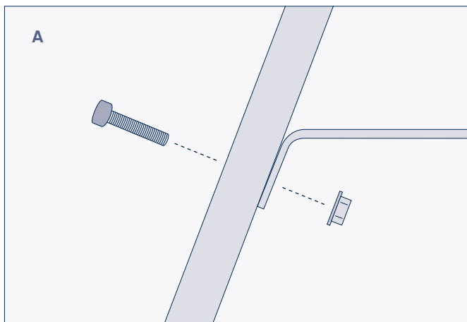
A: Die abgewinkelte Seite des Aufstellwinkel zeigt vom Balkon weg.
