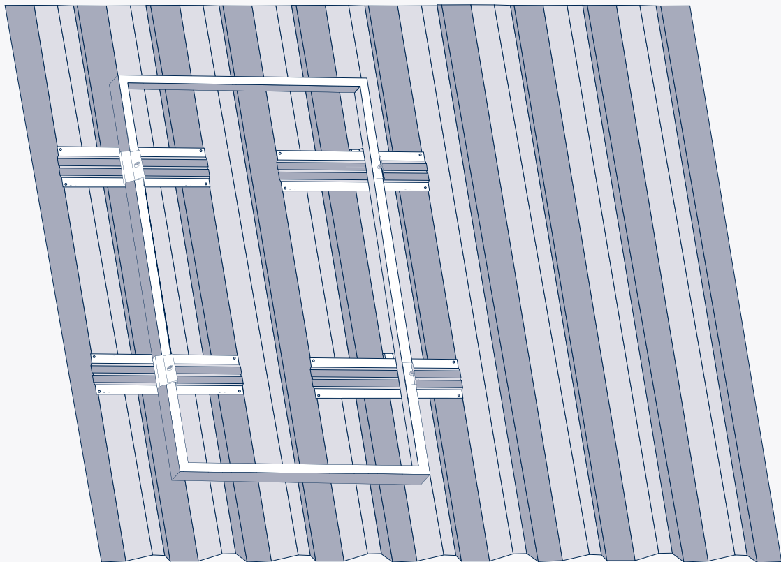
1. Nutenstein eindrücken
