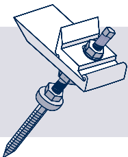
2 × Stockschrabe M10 × 180
