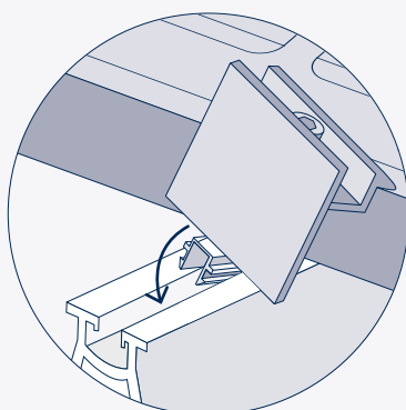
1. Nutenstein einschwenken
