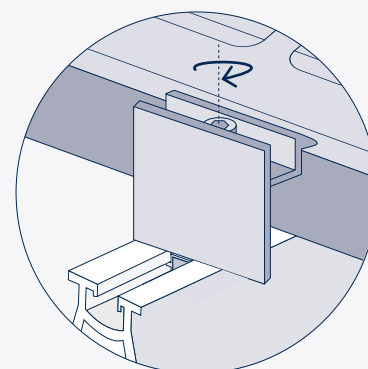
3. Festschrauben
