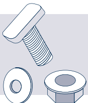
05 Hammerkopfschraube M8 × 25 mit Scheibe und Mutter
