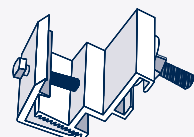
10 Wechselrichterhalterung (inkl. Hammerkopfschraube M8 x 25 mit Scheibe und Mutter)
