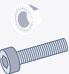
04 Nur mit Aufstellwinkel: Innensechskantschraube 2 × M8 x 40 mit Mutter
