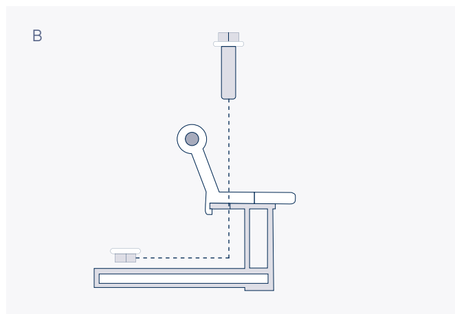
B: Der Haltepunkt des Scharniers zeigt nach Innen , in das Solarmodul.
