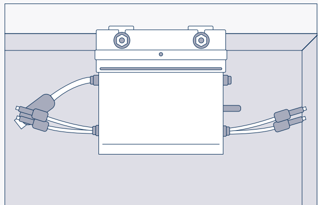
600 W - Wechselrichter
