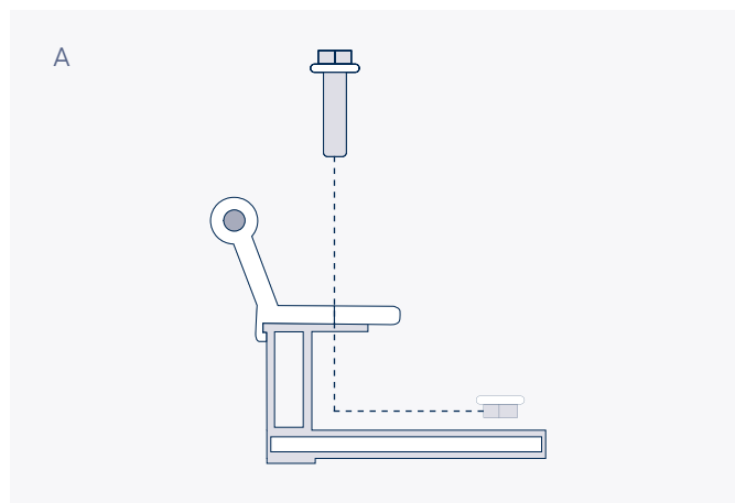
A: Der Haltepunkt des Scharniers zeigt nach Außen
